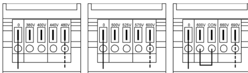
Изображение 4-5 Установочные клеммы для трансформатора вентилятора (3 AC 380–480 В / 3 AC 500–600 В / 3 AC 660–690 В)
