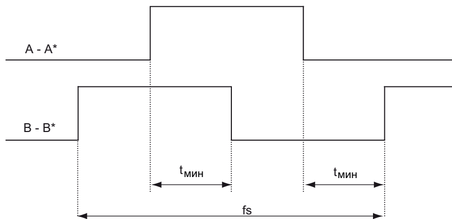
Изображение 4-37 Характеристика сигнала дорожки A и B между двумя фронтами: Время между двумя фронтами для импульсных датчиков
