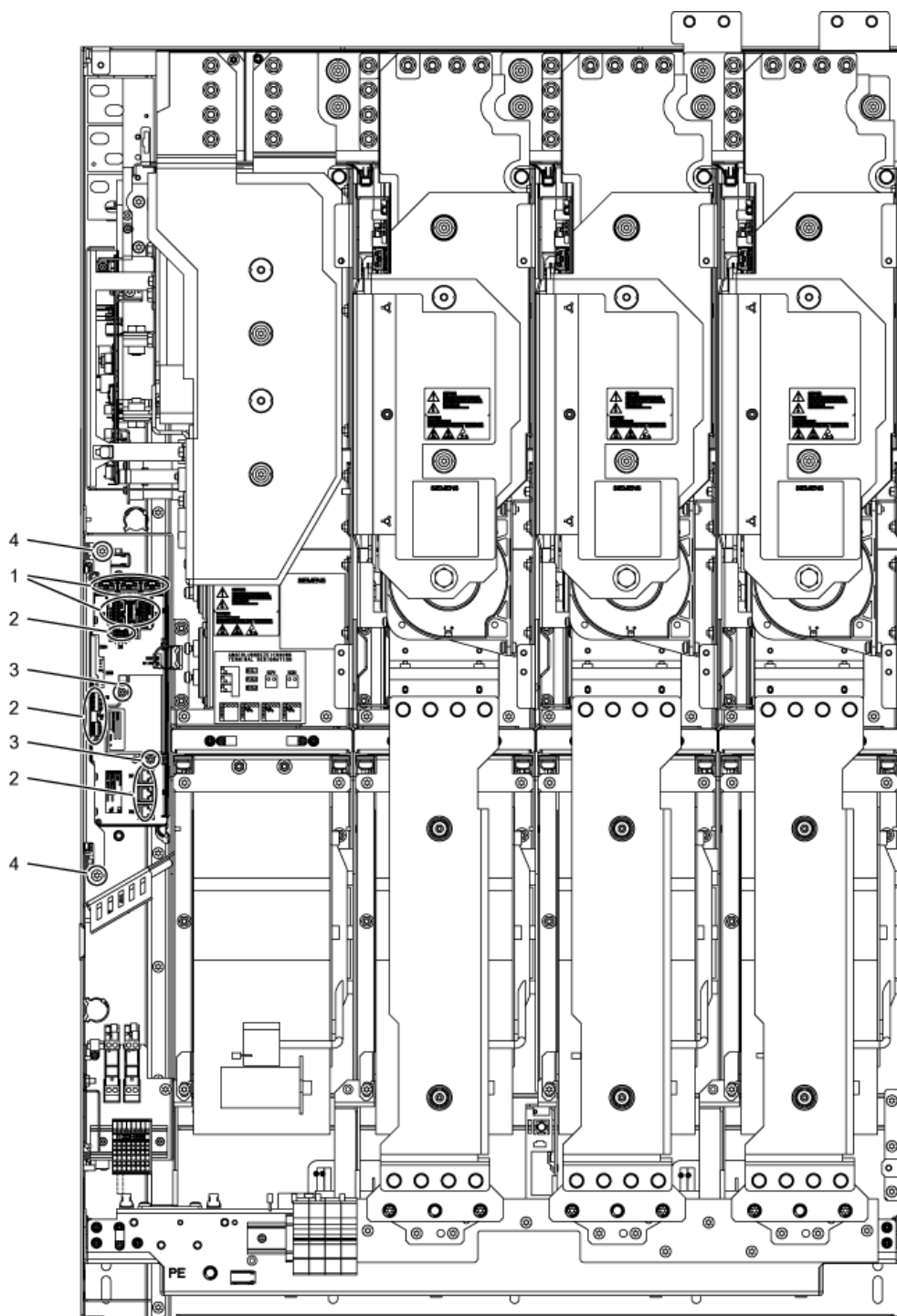
Изображение 11-7 Замена интерфейсного модуля управления, типоразмер JX
