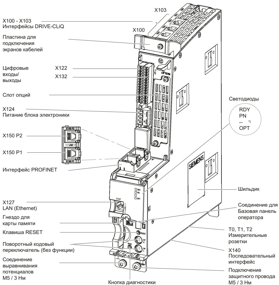
Изображение 4-47 Обзор соединений управляющего модуля CU320-2 PN (без крышки)
