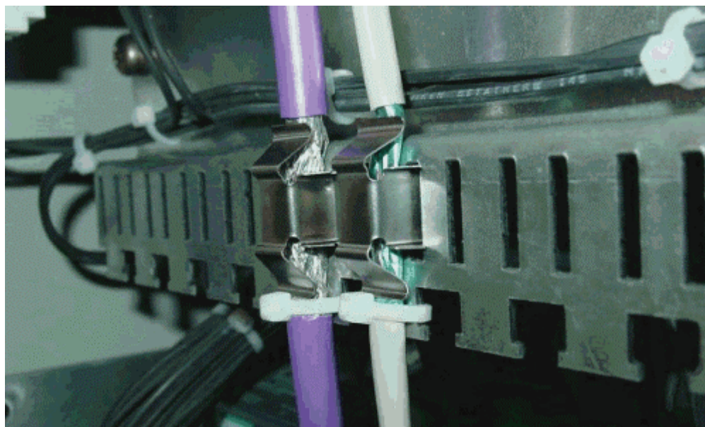
Изображение 4-16 Опора для экрана
