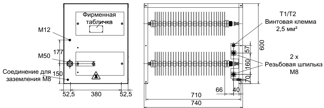
Изображение 4-21 Габаритный чертеж тормозного резистора 25 кВт
