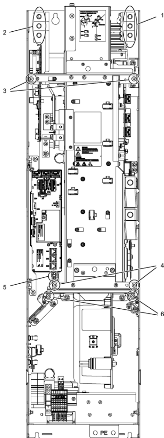
Изображение 11-8 Замена силового блока, типоразмер FX
