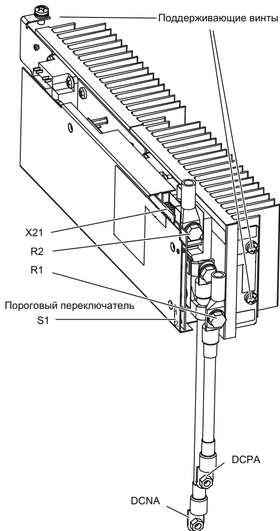
Изображение 4-25 Тормозные модули типоразмера GX
