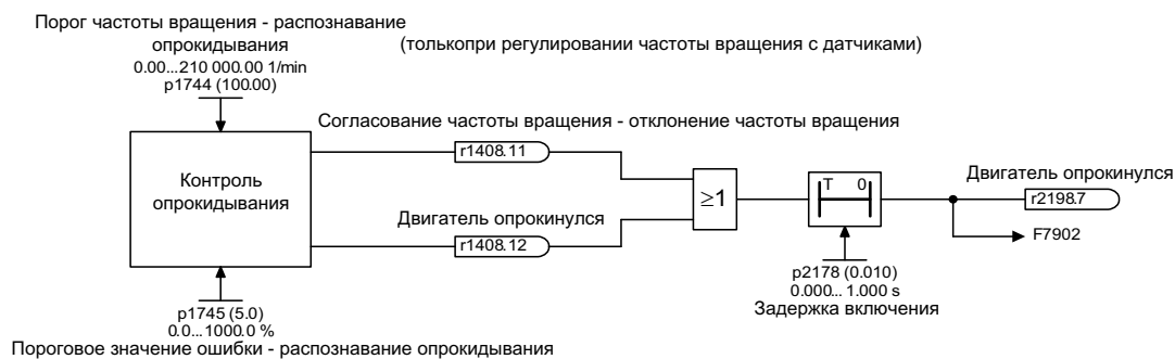
Изображение 9-19 Защита от опрокидывания
