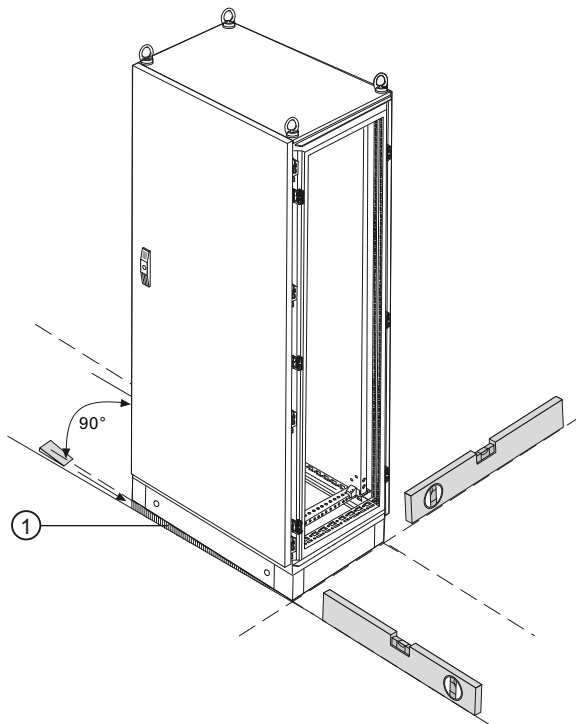
Изображение 3-1 Требование плоскостности основания
