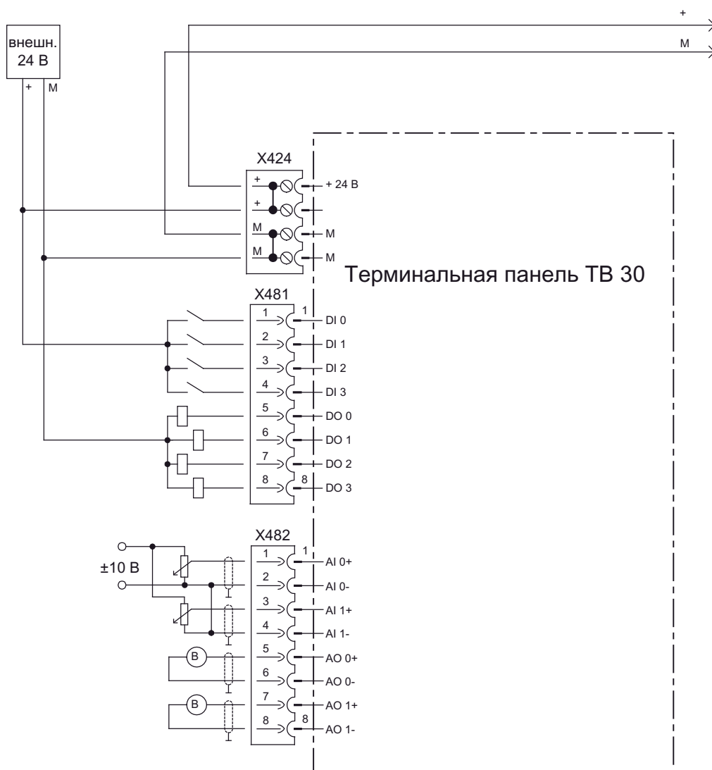
Изображение 4-45 Обзор соединений - терминальная плата ТВ30
