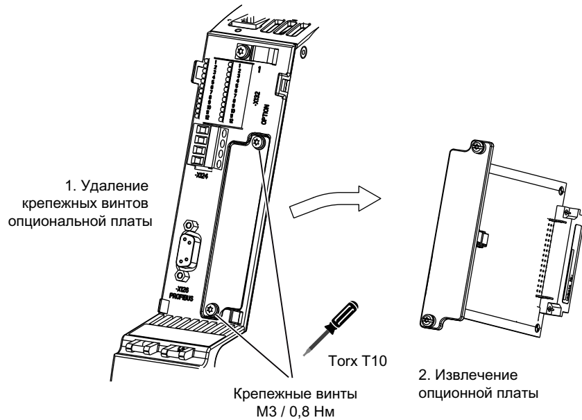
Изображение 4-32 Демонтаж CBE20 из слота опций управляющего модуля
